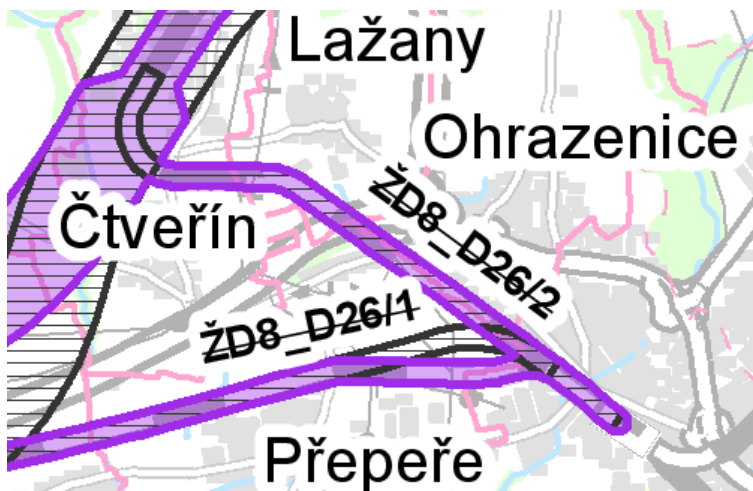
Obr. 3 Rušené narovnání trati na hranicích obcí Přepere, Turnov, Ohrazenice (zvětšený výřez z výkresu ploch a koridorů včetně ÚSES)
